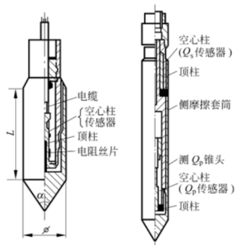
图1 双桥静力触探试验
