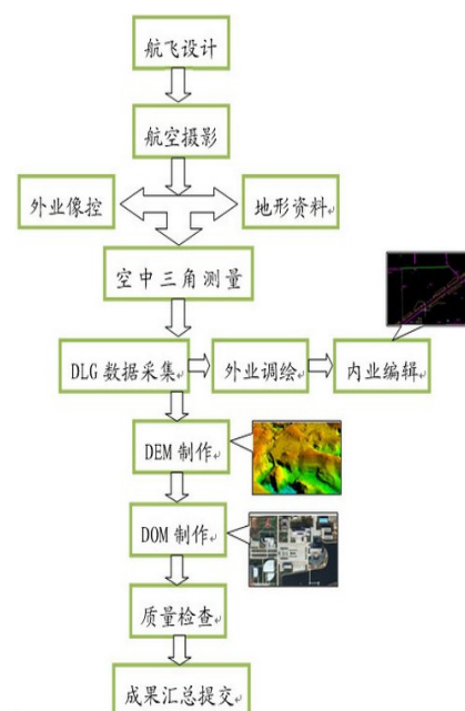
图1 无人机航空摄影测量技术流程图
